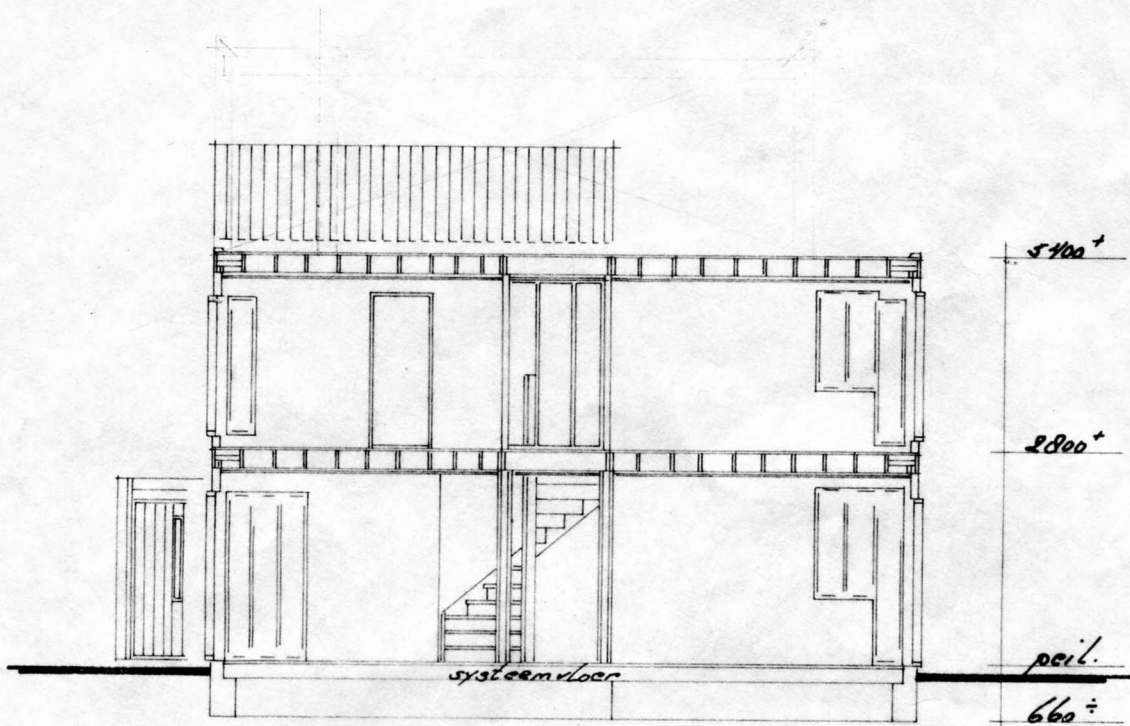
doorsnede A-A
