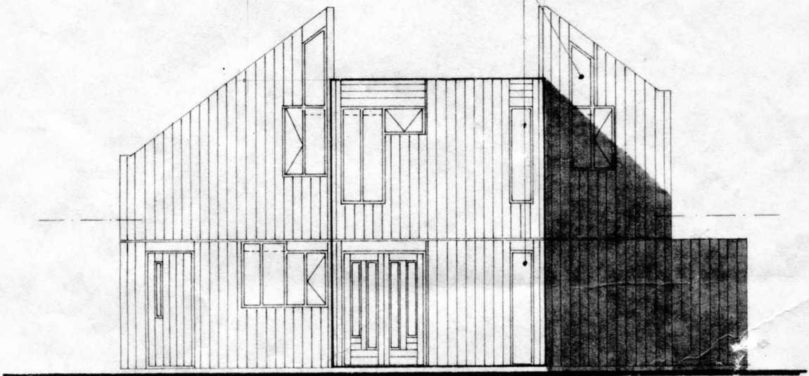
achtergevel woningtype 4a
