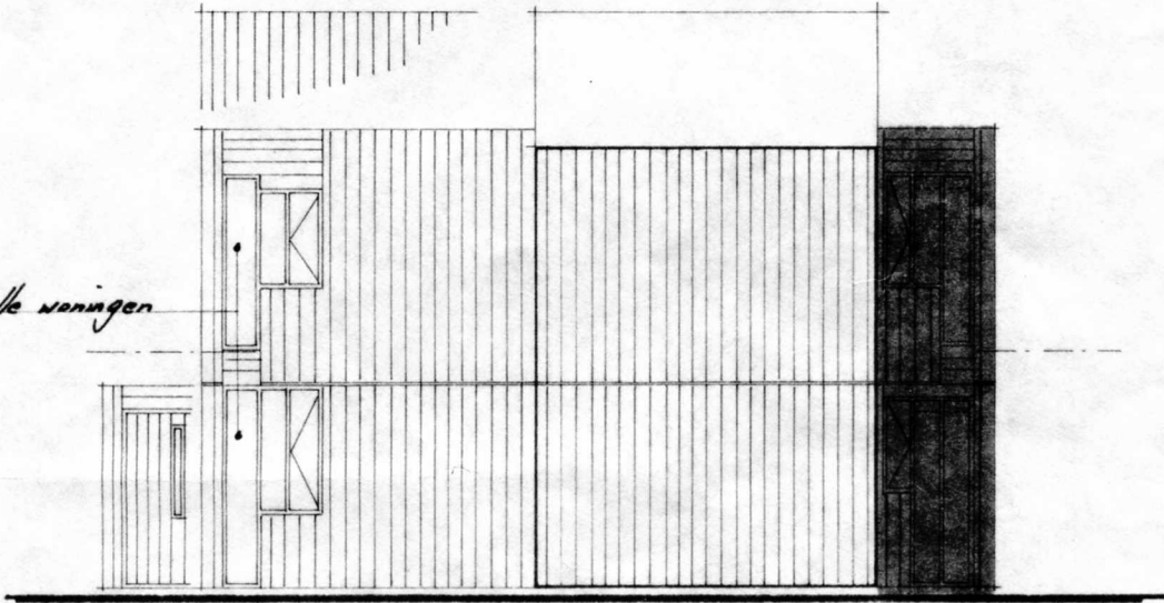
rechter zijgevel woning type 4 1/2
