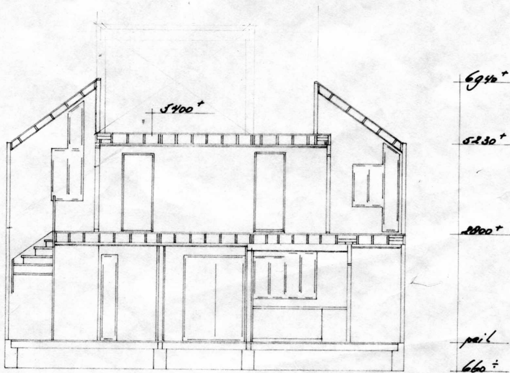
doorsnede B-B
